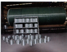
连续缠绕加强玻璃纤维筒体，计算机控制缠绕工艺，确保厚度均匀并达到设计要求质量稳定优良
